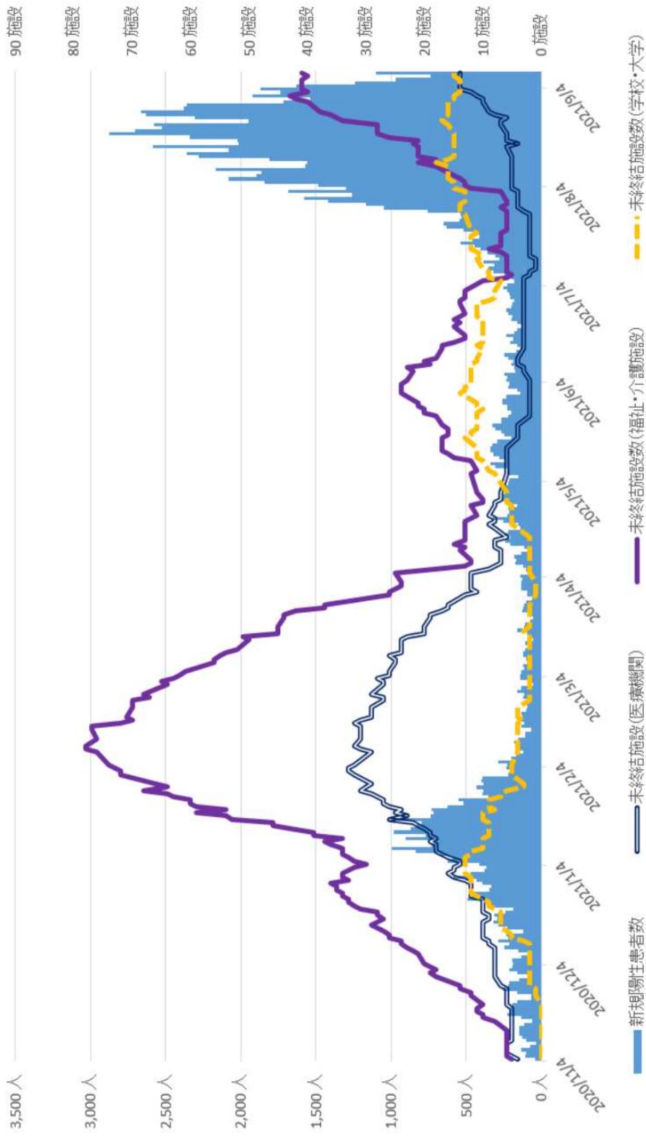
新規陽性患者数とクラスター未終結施設数
