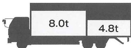
大型トラック
