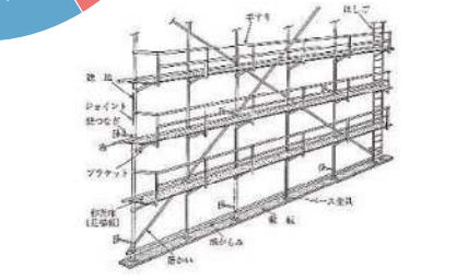
一側足場の例((一社)仮設工業会より提供)
