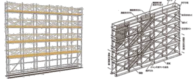
本足場の例((一社)仮設工業会より提供)
